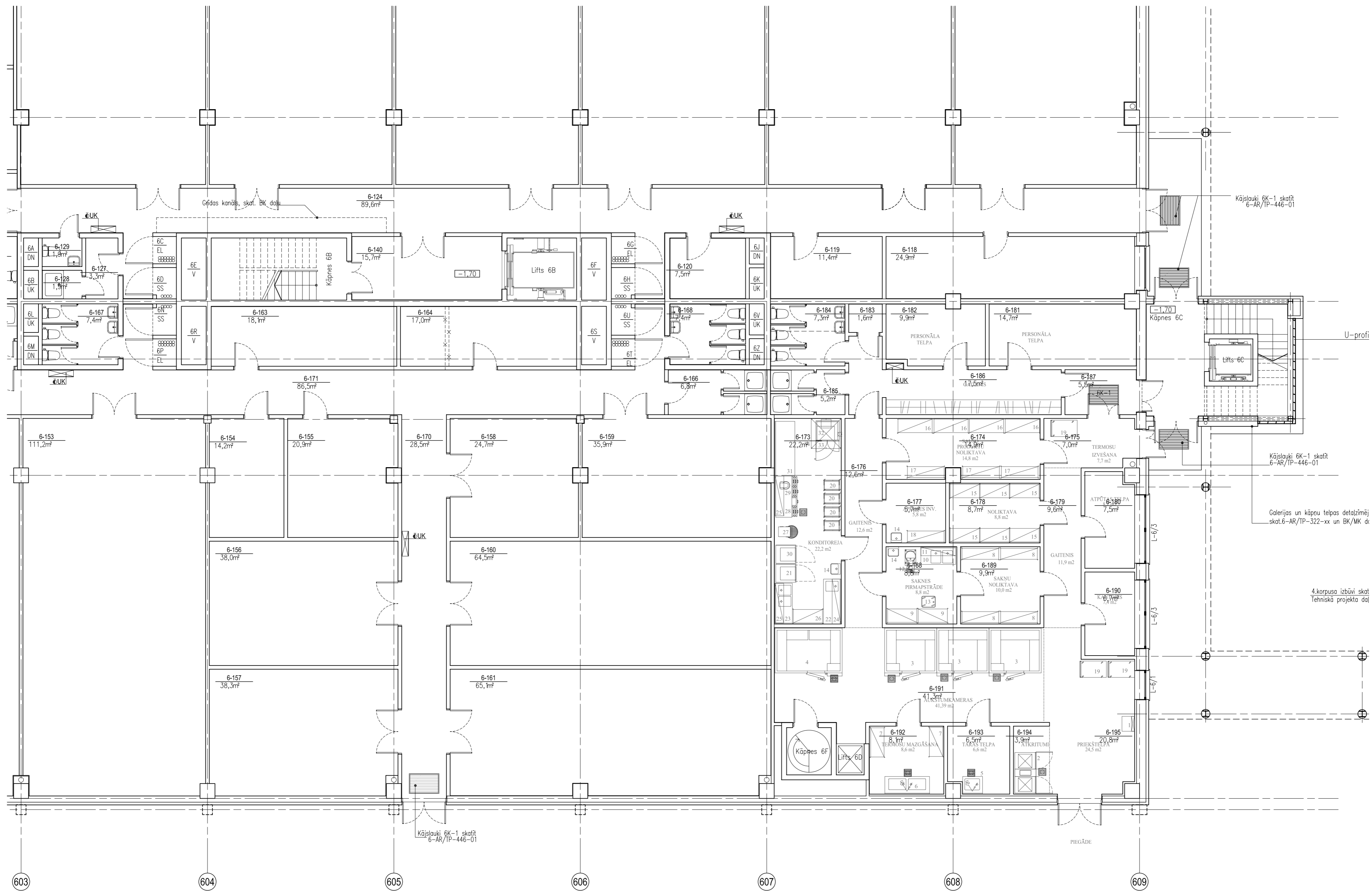
6.KORPUSA 1.STĀVA PLĀNA FRAGMENTS MĒROGS 1:100
